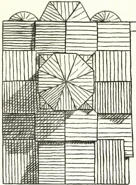
Εἰκ. 10. Λιτῆρες τῆς στέγης (σχέδιον H. Schleif).
