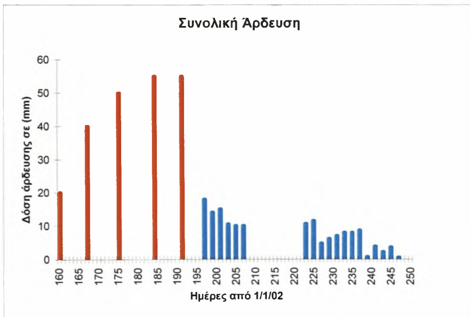
Σχήμα 5.2. Δόσεις άρδευσης καρποφορίας με σταγόνα.
