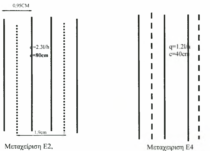
Διάταξη σταλακτηφόρου σωλήνα
