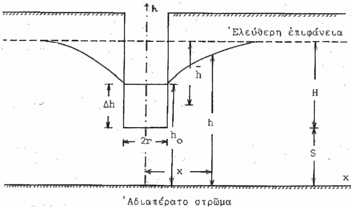
ΣΧΗΜΑ 2.2. Μέτρηση για την περίπτωση υπάρξεως ελεύθερης επιφάνειας
