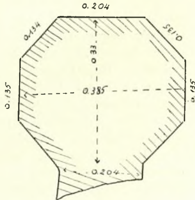
Εἰκ. 10. Τομὴ στύλου ἐνουμένου μετὰ τοίχου.
