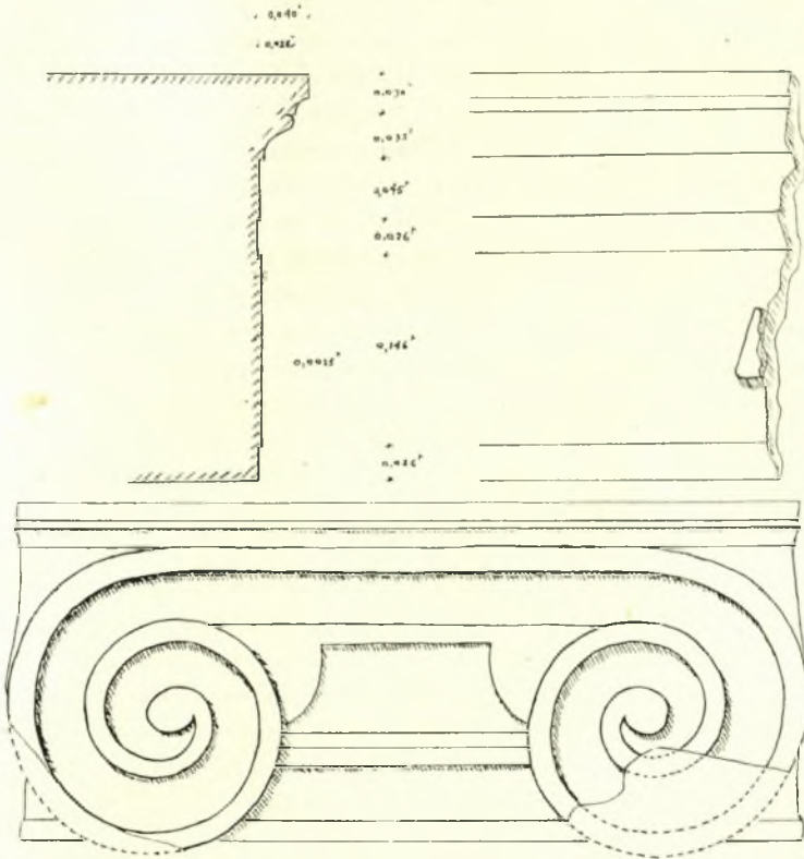
Εἰκ. 3. ἄνω. Ἐπίκρανον παραστάδος· κάτω σχέδιον Ἰωνικοῦ κονοκράνου εἰκ. 2.
