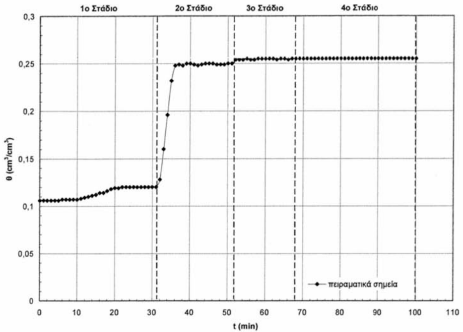
Σχήμα 4.18 Εδαφική υγρασία σε συνάρτηση με το χρόνο, κατά τη 2 η διύγρωση [Αμμώδες έδαφος (S)]
