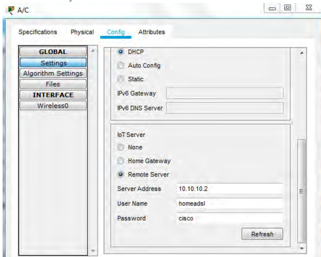
Παράδειγμα του IoT setup του Air Condition
