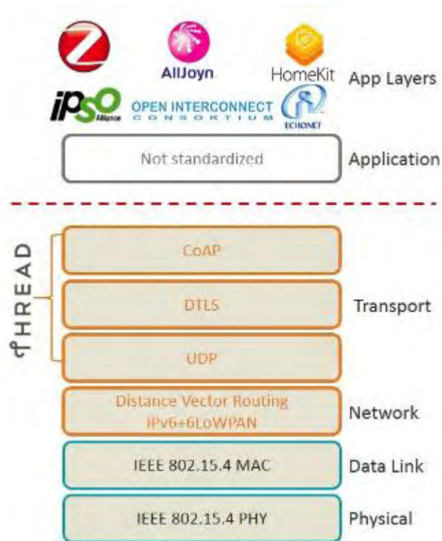
Η στοίβα πρωτοκόλλων του Thread [144]
