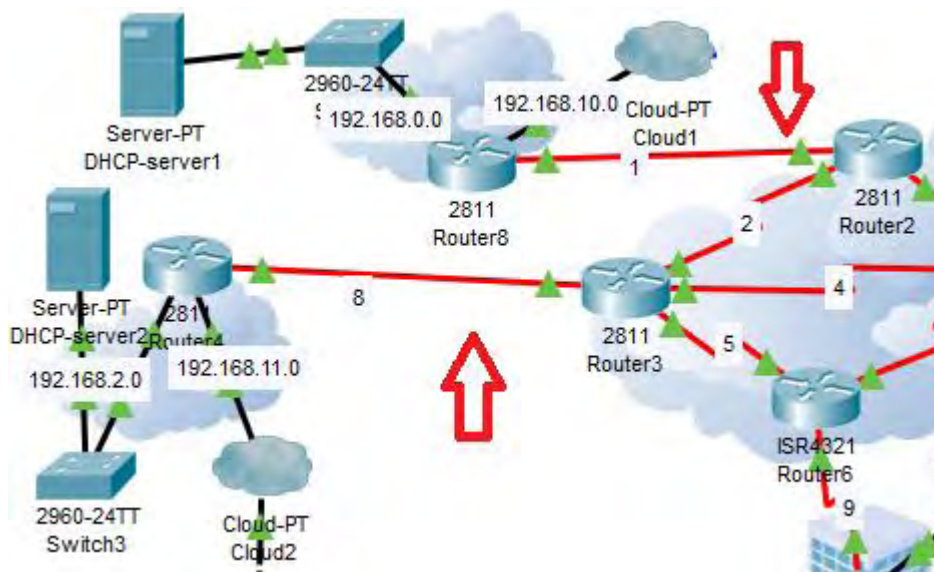
Fiber καλωδίωση μεταξύ των router στην προσομοίωση
