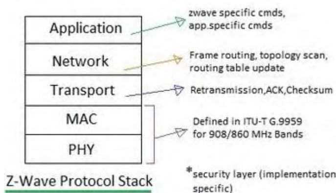
Στοιβα πρωτοκόλλου Z-Wave [142]
