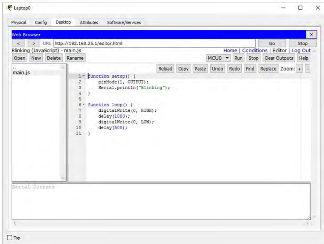
Παράδειγμα προγραμματισμού της πλακέτας MCU σε JavaScript (Packet Tracer) [50]
