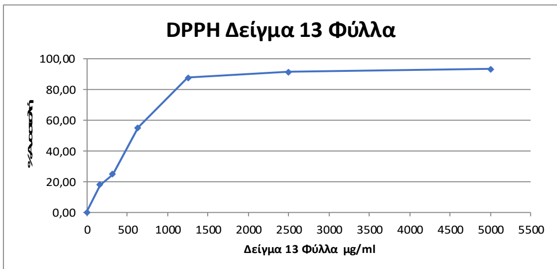
Διάγραμμα 12. Το διάγραμμα απεικονίζει την % αναστολή (εξουδετέρωση) της ρίζας DPPH από το εκχύλισμα Δείγμα 12 Φύλλα.
