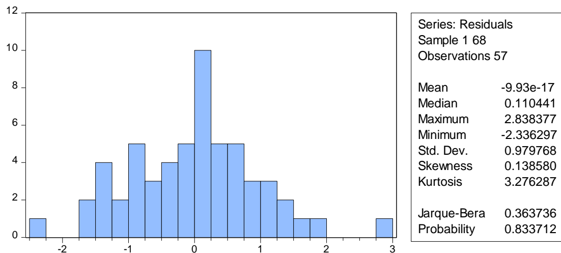
Γράφημα 7. Ιστόγραμμα συχνοτήτων των καταλοίπων τελικού υποδείγματος του πρώτου ερευνητικού ερωτήματος.
