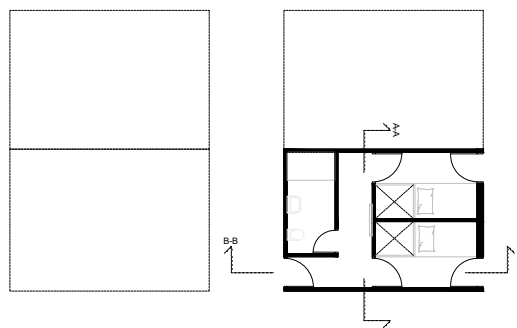
ΜΟΝΑΔΑ 2 ΑΤΟΜΩΝ
