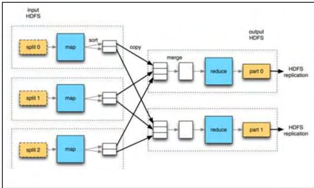
Εικόνα 8 : Τμήματα MapReduce
