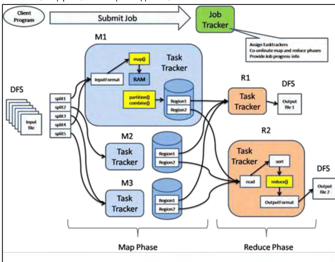
Εικόνα 7 : Αρχιτεκτονική MapReduce
