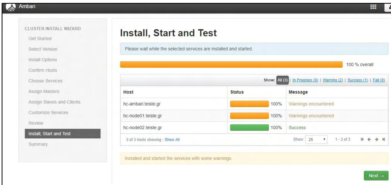
Εικόνα 22: Ολοκλήρωση εγκατάστασης
