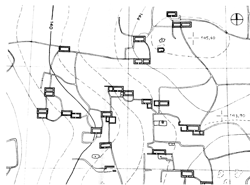
τοποθέτηση των κατασκευών κάθετα στις υψομετρικές καμπύλες (πηγή: Γ. Σαΐτας, Ελληνική Παραδοσιακή Αρχιτεκτονική)
