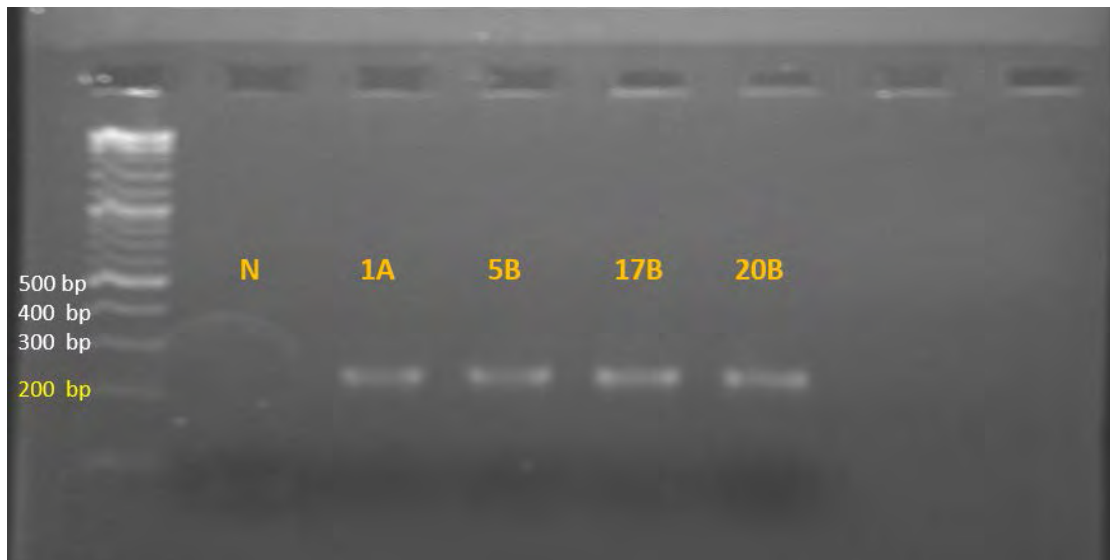
Εικόνα 11 Ηλεκτροφόρηση σε πηκτή αραρόζης 1% PCR προϊόντων εσωτερικής ένδεσης του γονιδίου 16S rRNA (περίπου 200 bp). Το N αντιστοιχεί στον αρνητικό μαρτυρα της αντίδρασης. Θετικό προϊόν και για τα 4 δείγματα
