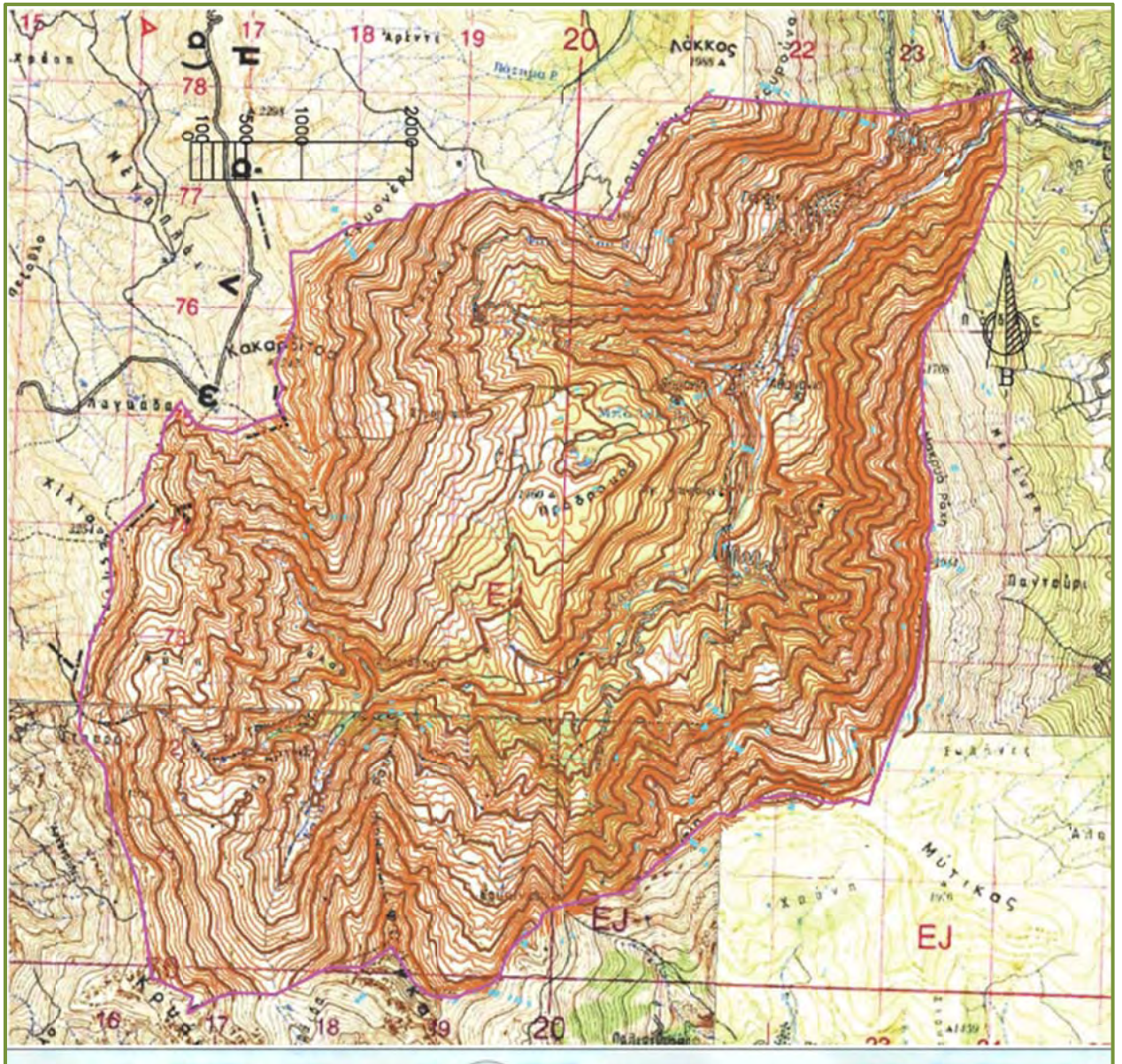
Σχήμα 4.3: Οι κύριες και οι ενδιάμεσες ισοψείς καμπύλες της λεκάνης απορροής
