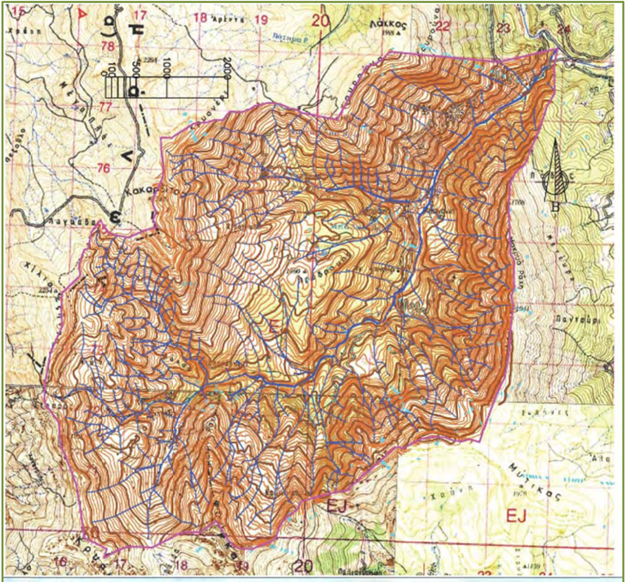
Σχήμα 6.1: Ο τελικός χάρτης της λεκάνης απορροής του χειμάρρου Μουτσιαρίτη μετά τον επαναπροσδιορισμό.
