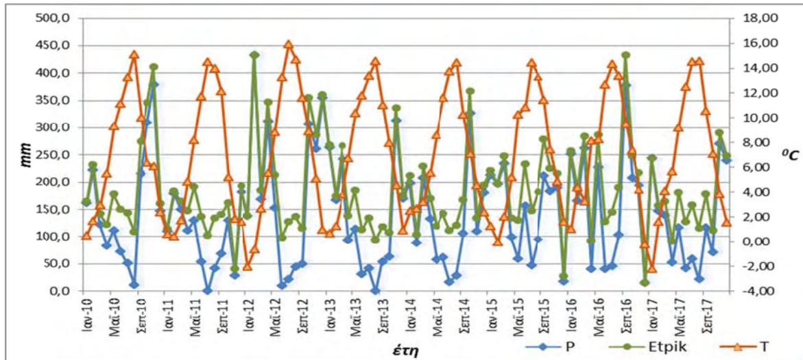
Σχήμα 6.8: Η βροχόπτωση, η θερμοκρασία και εξατμισοδιαπνοή στη λεκάνη απορροής του χειμάρρου Μουτσαρίτη για τη χρονική περίοδο 2010-2017
