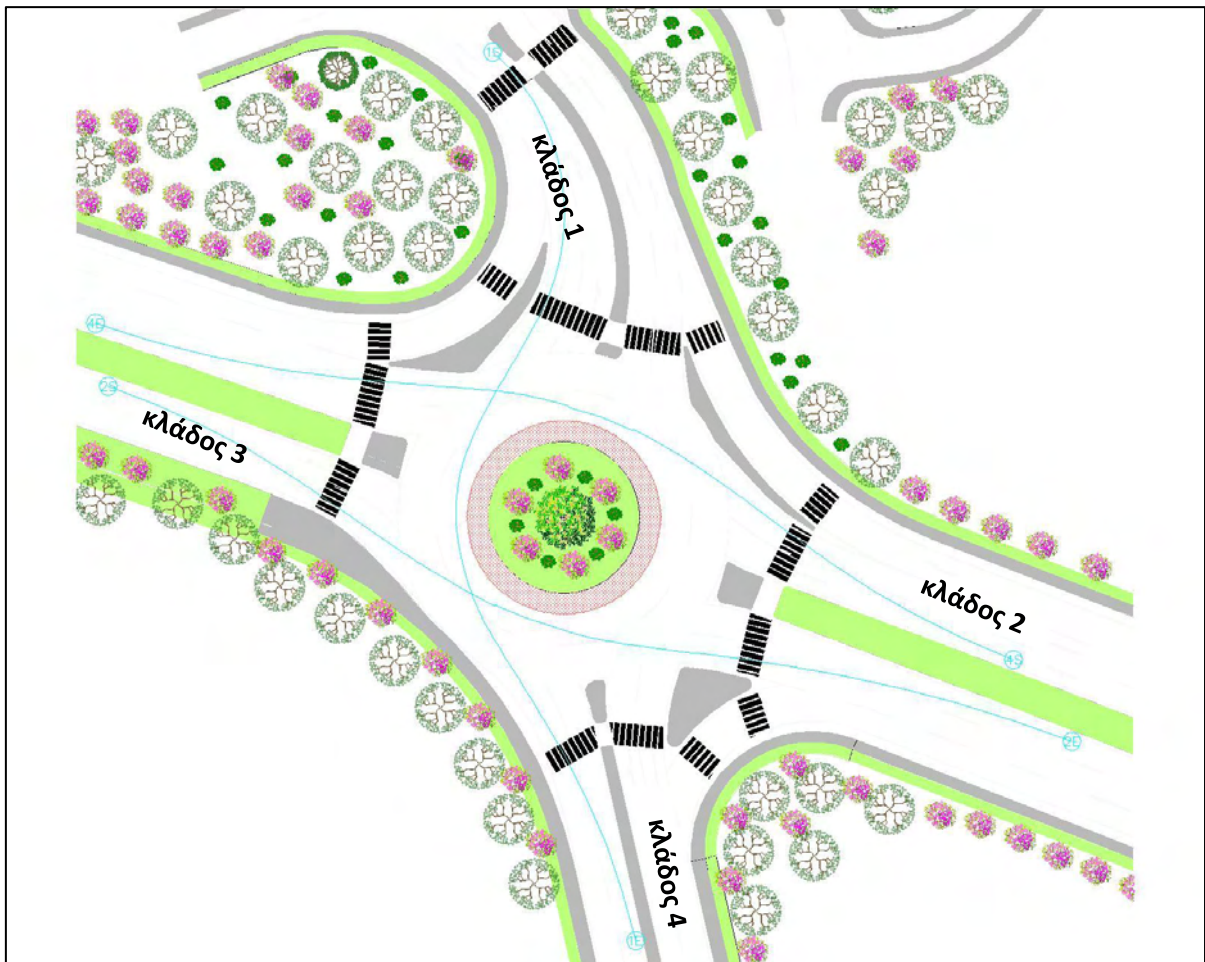
Διάγραμμα 8.7.1-1 Πορείες οχημάτων κατά την εκτέλεση της συντομότερης διαδρομής για την εκτίμηση των ταχυτήτων που αναπτύσσονται στον κόμβο.
