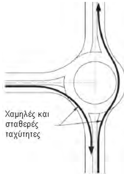
Σχήμα 3.2.5-2 Γωνίες μεταξύ των κλάδων προσέγγισης σε διασταύρωση διάταξης «Τ» (National Cooperative Highway Research Program, 2010 και ίδια επεξεργασία)
