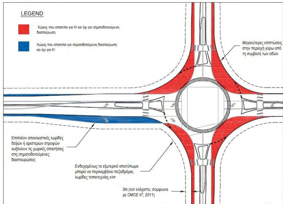
Σχήμα 2.3.2-1 Σύγκριση χωρικών απαιτήσεων ενός K^3 μία λωρίδας έναντι συγκρίσιμης σηματοδοτούμενης διασταύρωσης (NCHRP & FHWA, 2010, Ίδια Επεξεργασία).
