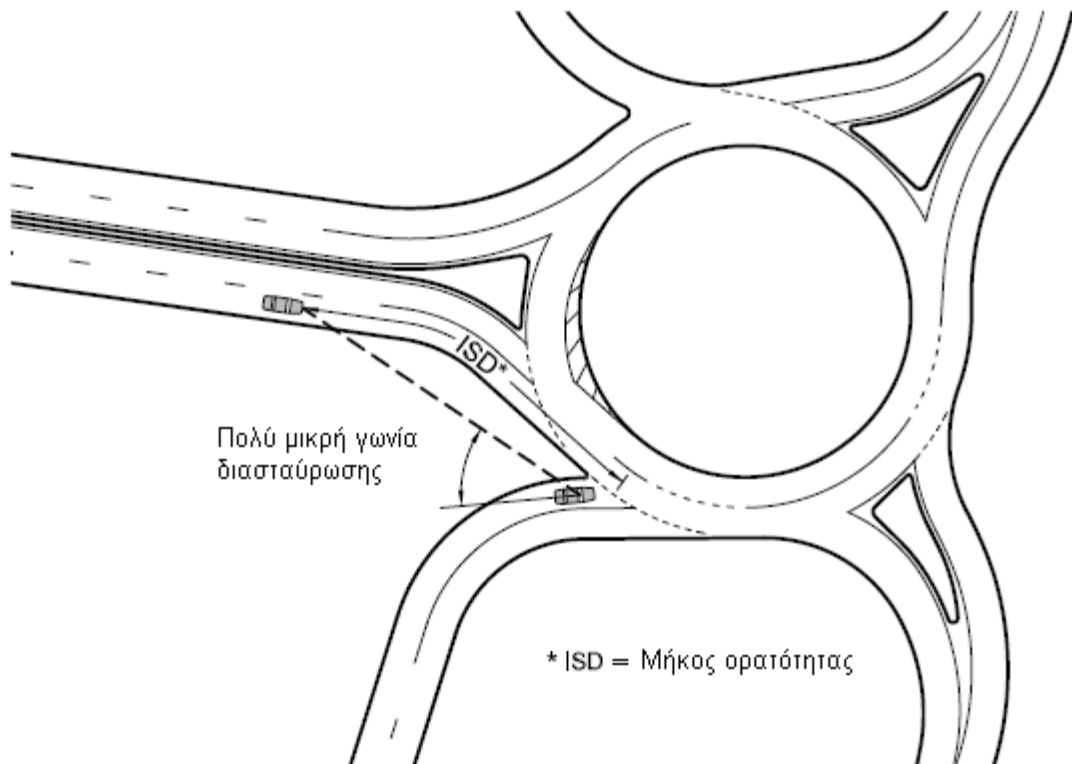
Σχήμα 3.3.3-5 Παράδειγμα σχεδιασμού με πολύ μικρή γωνία ορατότητας προς τα αριστερά (<math><75^\circ</math>), Πηγή: National Cooperative Highway Research Program, 2010 και ίδια επεξεργασία
