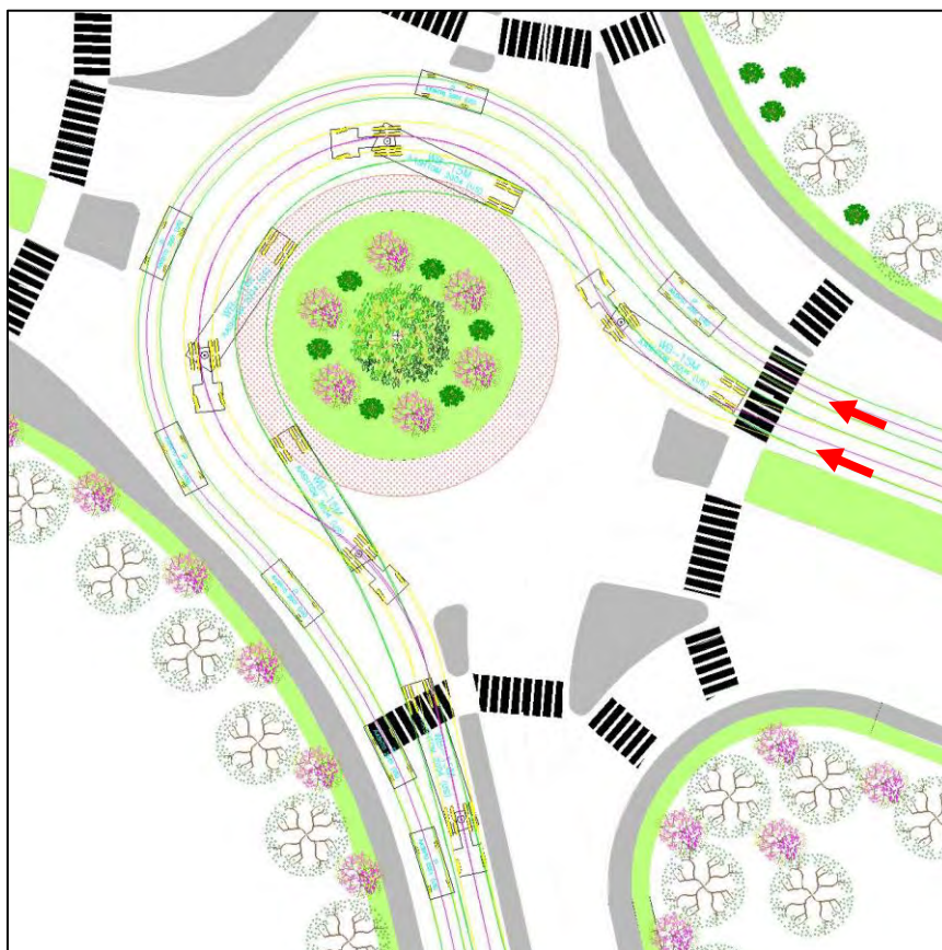
Διάγραμμα 8.7.4 – 2 Κίνηση Ανατολή – Νότος του οχήματος σχεδιασμού (WB-15) παράλληλα με Ι.Χ. (μεγάλος κυκλικός κόμβος)
