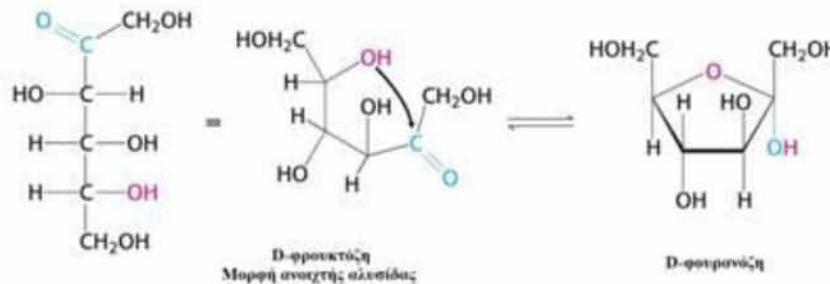
Εικόνα 3: Σχηματισμός φουρανόζης
