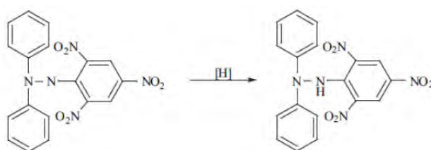
Εικόνα 15: Η αναγωγή του DPPH• σε DPPH:H
