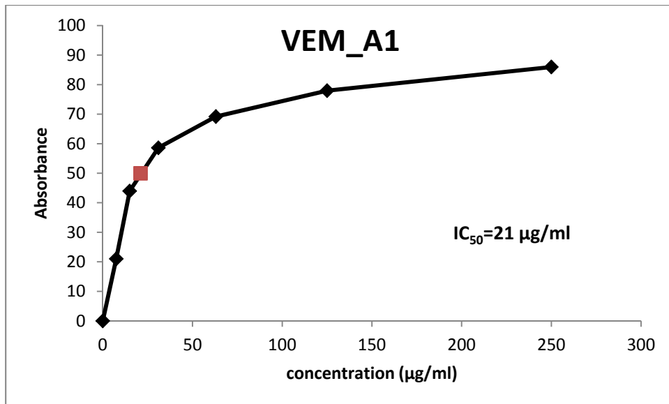
Διάγραμμα 12: Η % αναστολή της ρίζας O_2^- \bullet από το εδώδιμο χόρτο VEM_A1.
