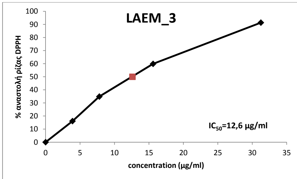
Διάγραμμα 2: Η % αναστολή της ρίζας DPPH από το εκδόδιμο χόρτο LAEM_3
