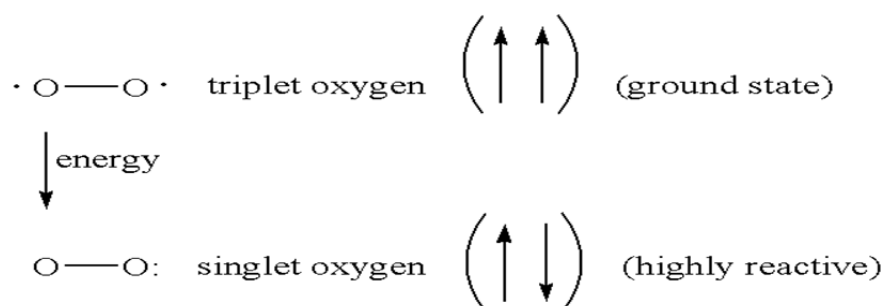
Εικόνα 2: Οξυγόνο μονής και τριπλής κατάστασης
