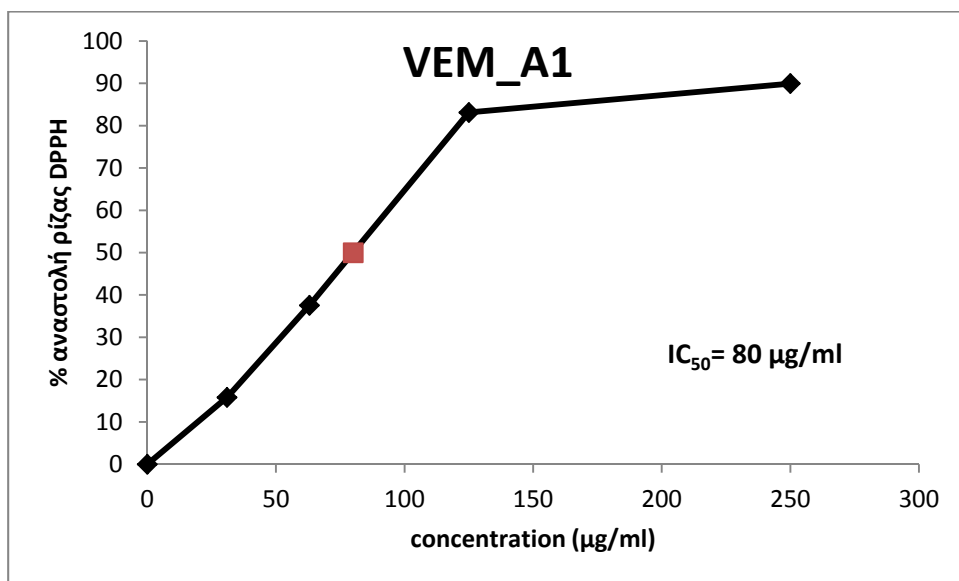
Διάγραμμα 3: Η % αναστολή της ρίζας DPPH από το εκδόδιμο χόρτο VEM_A1
