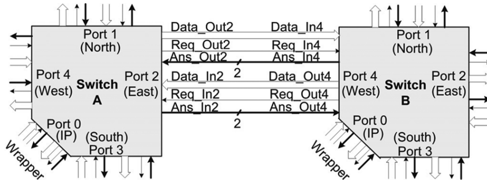
Εικόνα 5.7 Switch-by-Switch διασύνδεση
