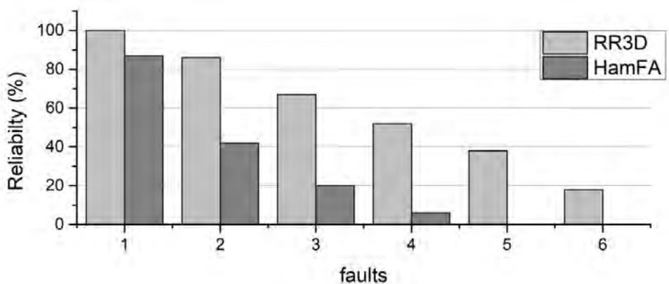
Εικόνα 20 Αξιολόγηση αξιοπιστίας σε α) Δίκτυο 2D, β) Δίκτυο 3D
