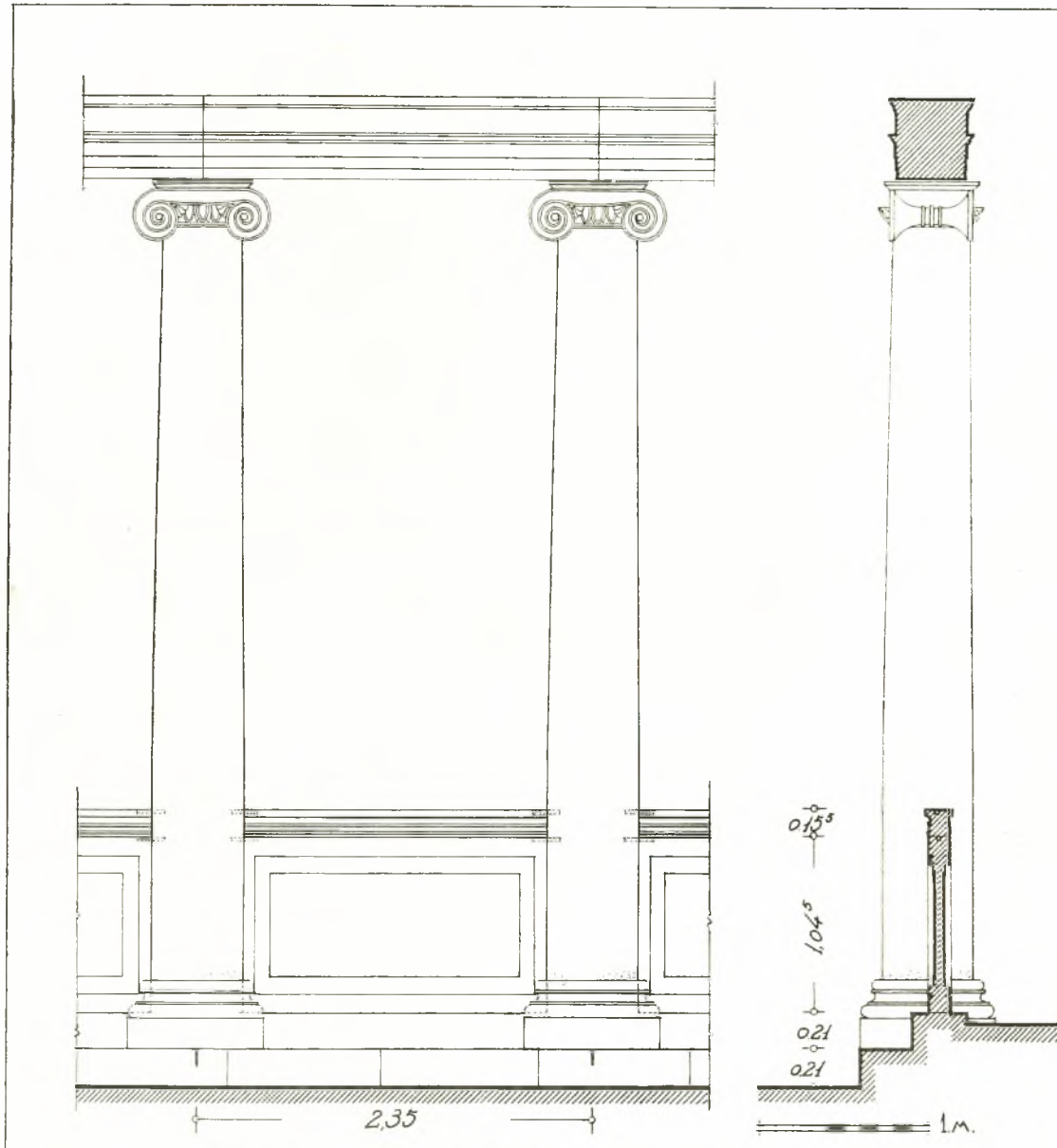
Εἰκ. 6. Ἀναπαράστασις τμήματος τῶν κιονοστοιχιῶν τοῦ κυρίου ναοῦ.
