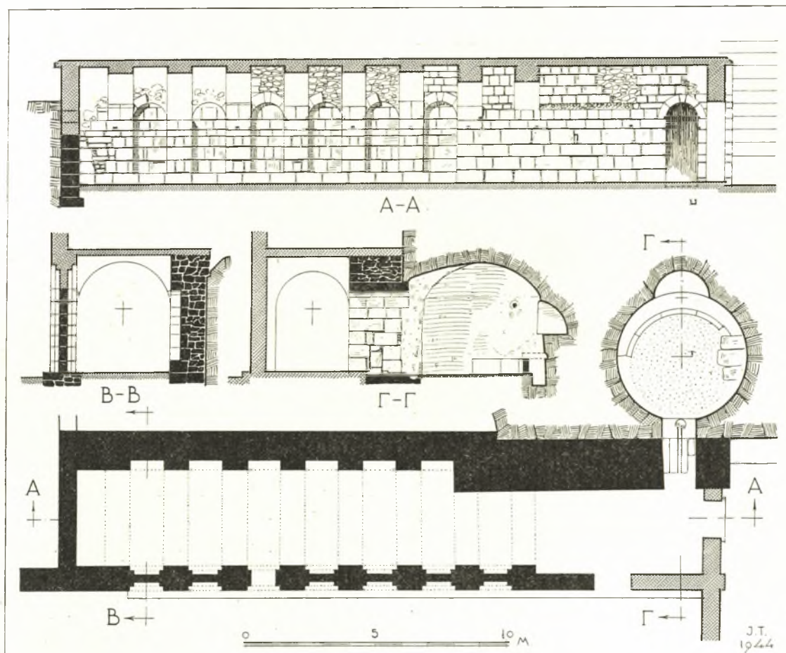
Εἰκ. 15. Κάτοψις τοῦ ἐπιμήκουσ οἰκοδομήματος καὶ τοῦ Ἀγιάσματος καὶ διάφοροι τομαί.
