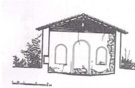
Εικόνα 23. Αγιά Λάρισα, Μονή Αγίου Παντελεήμονος, αρχιτεκτονικό σχέδιο της Τράπεζας.
