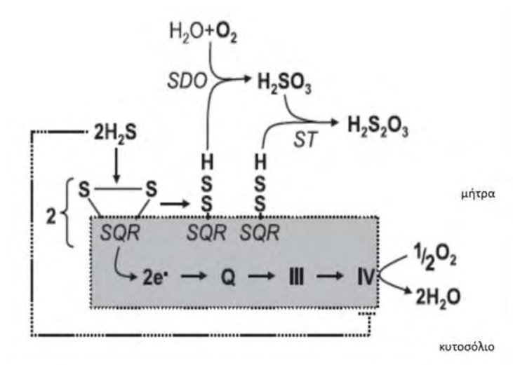
Εικόνα 16: Μιτοχονδριακή οξείδωση H_2S . Ανατύπωση από (Olson 2011).
