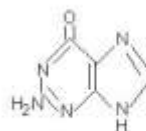
Γουανίνη
