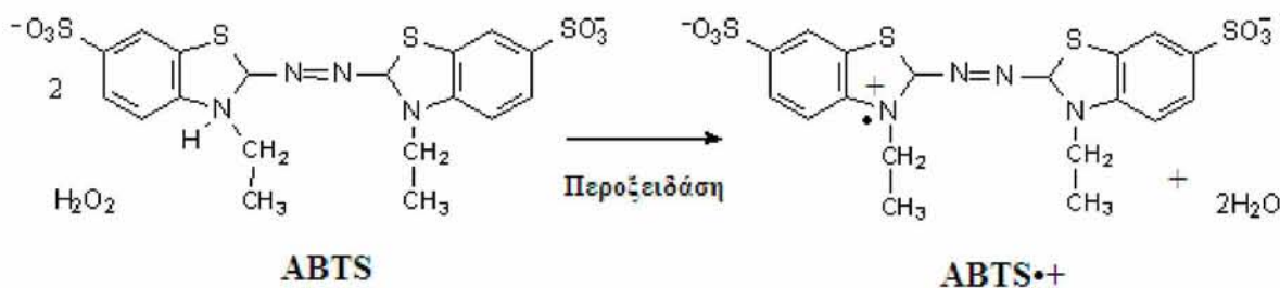
Εικόνα 40. Χημική δομή και ενζυμική παραγωγή της ρίζας ABTS •+ μέσω της δράσης της περοξειδάσης.
