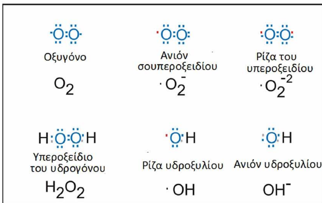
Εικόνα 1. Δραστικές Μορφές Οξυγόνου
