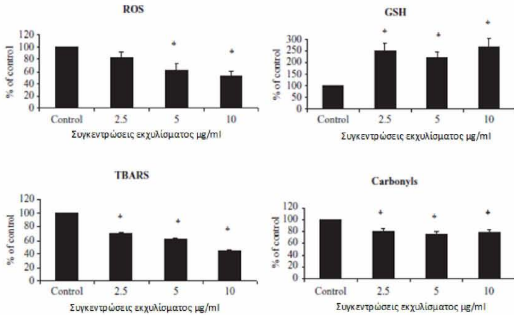
Εικόνα 25. Παρουσιάζεται η επίδραση της χορήγησης του εκχυλίσματος στεμφύλων στα επίπεδα των ROS, GSH, TBARS, και πρωτεϊνικών καρβονυλίων. Τα επίπεδα των TBARS και των πρωτεϊνικών καρβονυλίων εκτιμήθηκαν με φασματοφωτομετρικά. Όλες οι τιμές παρουσιάζονται ως μέσος όρος \pm SEM τριών ανεξάρτητων πειραμάτων. * p < 0.05 : στατιστικά σημαντική διαφορά σε σύγκριση με τα κύτταρα ελέγχου.
