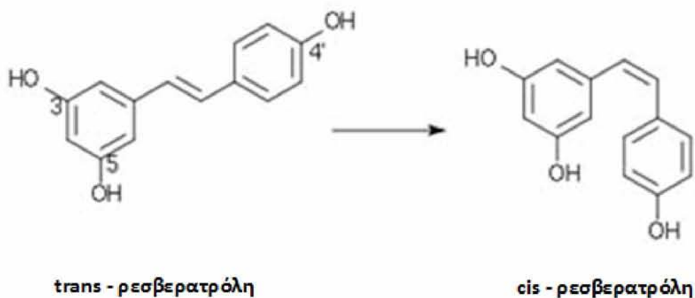
Εικόνα 12. Δομή trans και cis ρεσβερατρόλης
