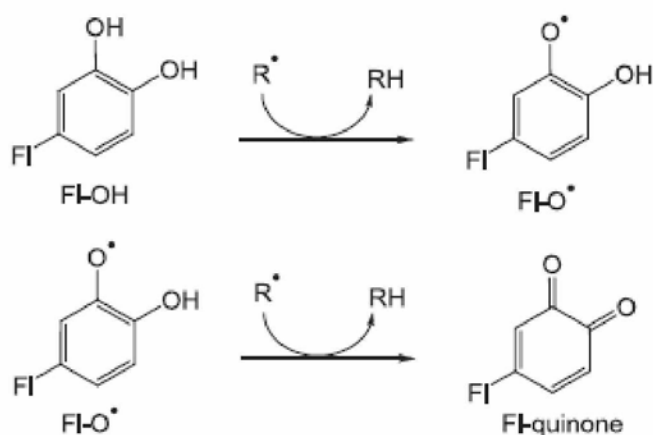
Εικόνα 14. Εκκαθάριση ελευθέρων ριζών ( \text{R}^\bullet ) από ένα φλαβονοειδές. Η ημικινόνη \text{FI-O}^\bullet αντιδρά με τη δεύτερη ρίζα αποκτώντας τη σταθερή δομή κίνησης.
