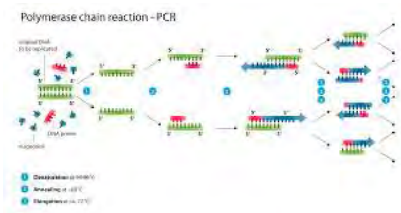
Εικόνα 16: Στάδια PCR
