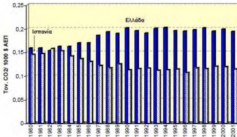
Σχήμα 2.8. Εξέλιξη της έντασης άνθρακα στην Ελλάδα για την περίοδο 1980-2001. Η κατανομή της κατανάλωσης ενέργειας και των εκπομπών CO2 ανά τομέα δραστηριότητας δίνονται στα διαγράμματα του Σχήματος 2.9, με τον τομέα των μεταφορών αυξάνει συστηματικά με τα χρόνια. Οι κατανομές αυτές είναι συγκρίσιμες με αντίστοιχες κατανομές στην Ε.Ε.
