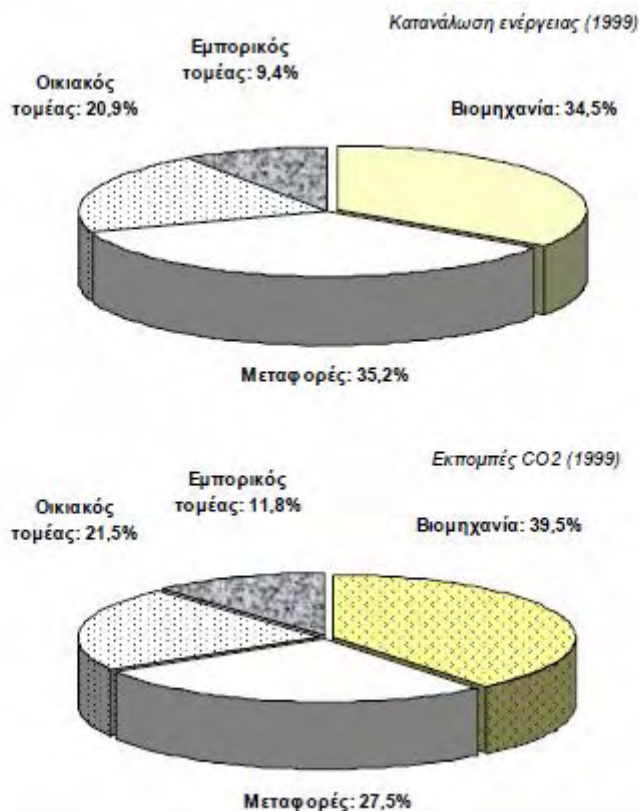
Σχήμα 2.9. Η συμμετοχή των διάφορων τομέων στην κατανάλωσης ενέργειας (επάνω) και στις εκπομπές CO 2 (κάτω) από την καύση ορυκτών καυσίμων στον κόσμο για το 2000.
