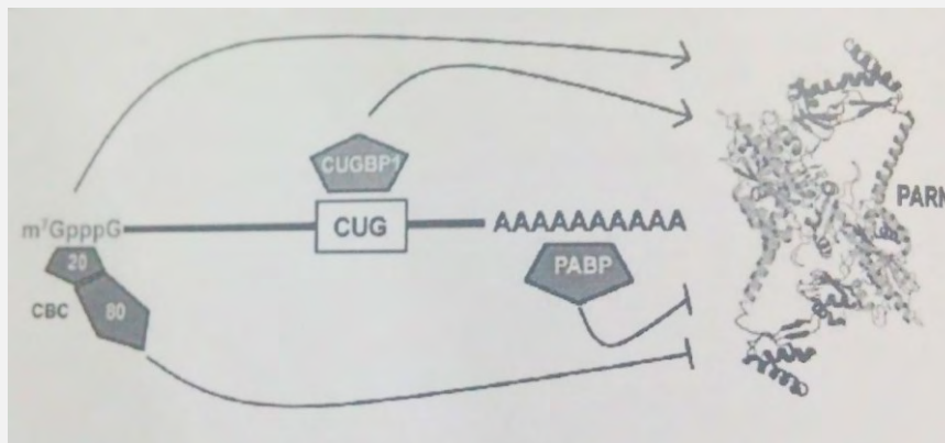
Εικόνα 6: Ρύθμιση της αποαδενύλασης μέσω από RNA-συνδεόμενων πρωτεϊνών (Virtanen et al.2013).
