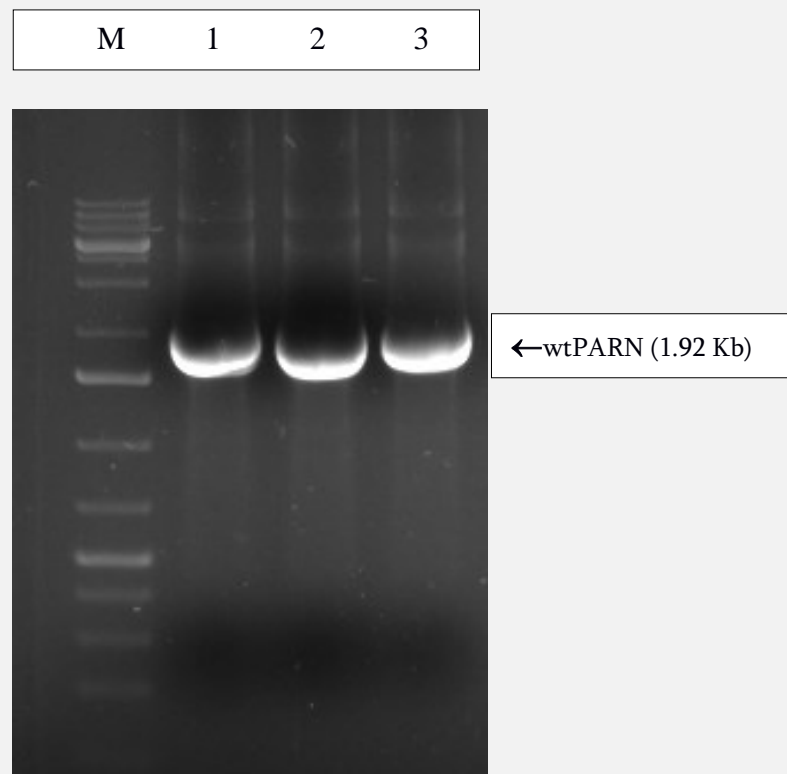
Εικόνα 17: Ηλεκτροφόρηση του προϊόντος PCR σε πηκτή αγαρόζης 1,5%. Διακρίνεται καθαρά η ειδική ζώνη στις 1,92kb που αντιστοιχεί στο cDNA της PARN. M: μάρτυρας DNA 1Kb. Διαδρομές 1,2,3: Προϊόντα ενίσχυσης PCR.
