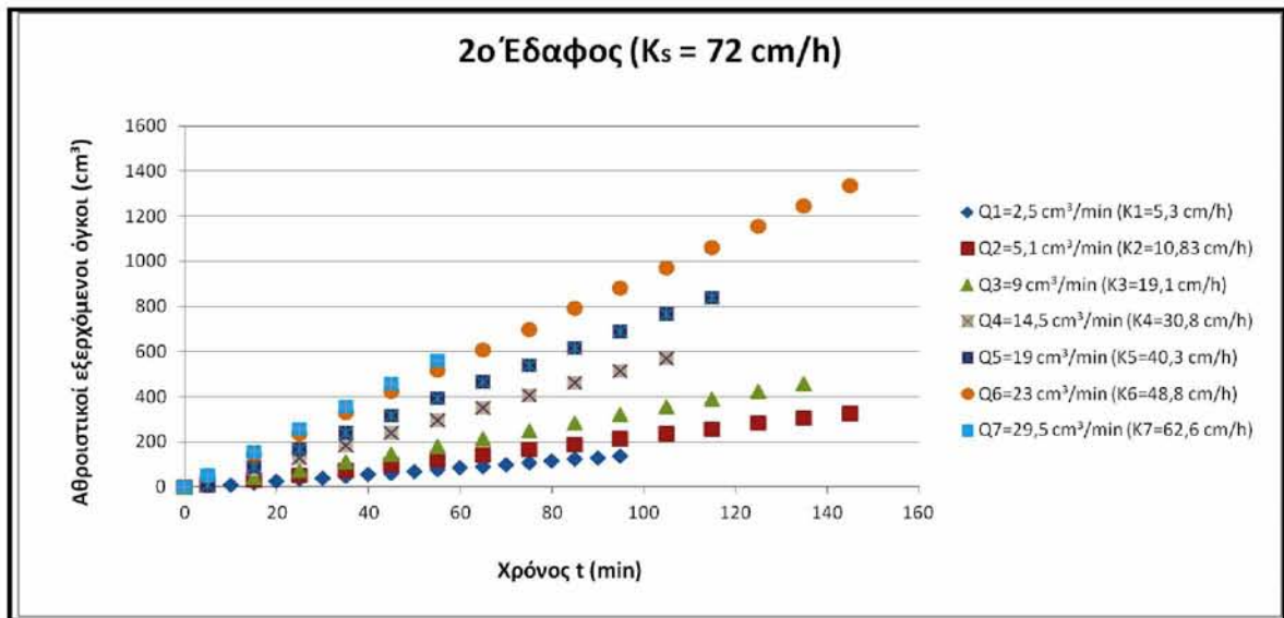
Διάγραμμα 37. Αθροιστικοί εξερχόμενοι όγκοι νερού (V) σε συνάρτηση με το χρόνο (t) για το δεύτερο εδαφικό δείγμα για όλες τις εφαρμοζόμενες παροχές.
