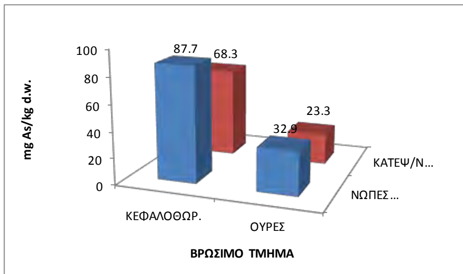
Σχήμα 4.12.: Συγκεντρώσεις As στον κεφαλοθώρακα και την ουρά, ειδών που αλιεύθηκαν εντός και εκτός Παγασητικού Κόλπου.
