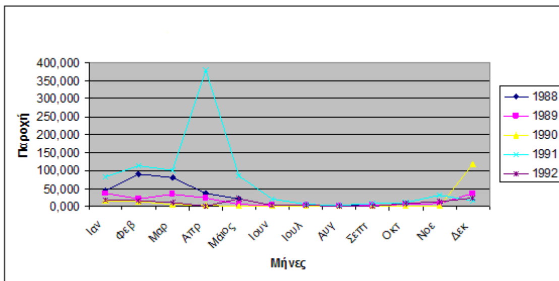
Σχήμα 30: Η παροχή του Πηνειού στη θέση Αγία Παρασκευή Τεμπών για τα έτη 1988-1992.
