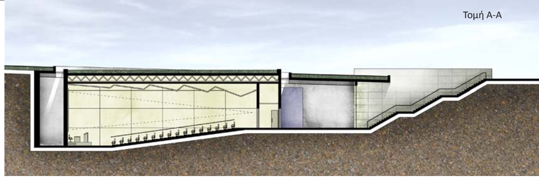
Τομή B-B
