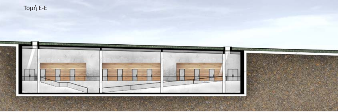
Τομή Z-Z
