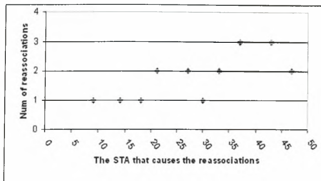
Σχήμα 5.5: Ο αριθμός των επανασυνδέσεων που η παρουσία ενός νέου σταθμού προκαλεί
