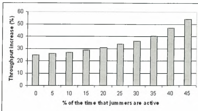
Σχήμα 5.4: Η αύξηση της ρυθμαπόδοσης κατά την παρουσία παρεμβολέων
