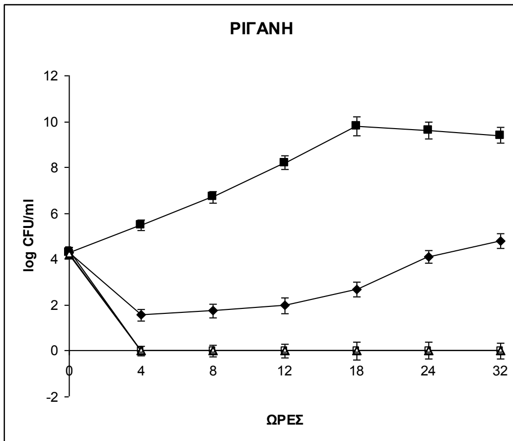
Σχήμα 6.1 Αντιμικροβιακή δράση του αιθέριου ελαίου ρίγανης κατά του V. parahaemolyticus in vitro στους 37 °C για 32 ώρες. (-■-) μάρτυρας, (-◆-) ρίγανη 0,2 %, (-△-) ρίγανη 0,4 %, (-□-) ρίγανη 0,6 %, (-○-) ρίγανη 0,8 %.
