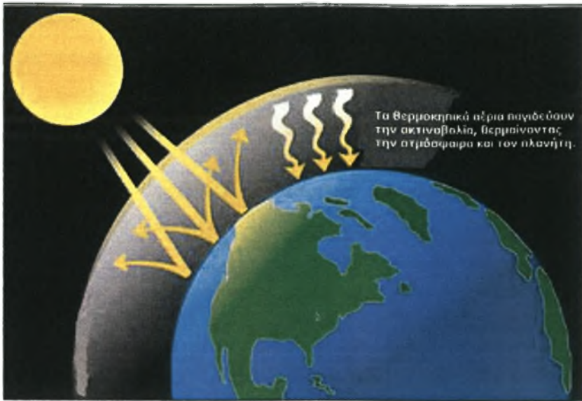
Εικόνα 2: Παγίδευση της ακτινοβολίας, φαινόμενο του θερμοκηπίου (www.europa.eu)
