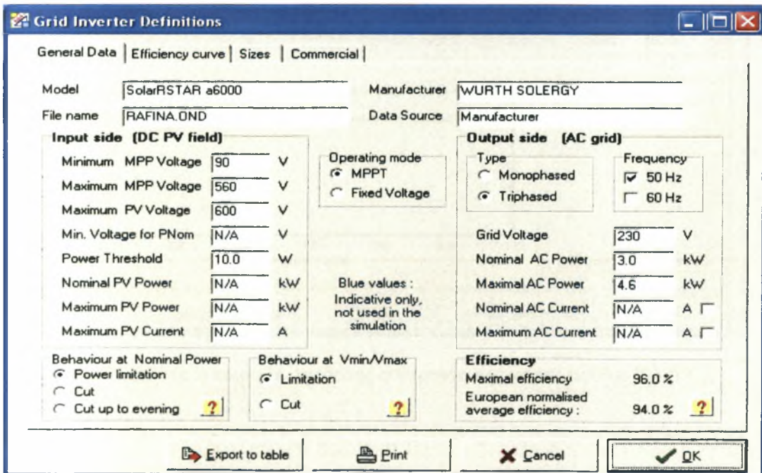
Εικόνα 35: Τεχνικά Χαρακτηριστικά
