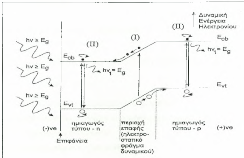
Εικόνα 6: Ηλιακό στοιχείο που αποτελείται από την επαφή ημιαγωγού τύπου-n και τύπου-p. Διάγραμμα της δυναμική ενέργειας των ηλεκτρονίων σε συνάρτηση με το βάθος από την επιφάνεια (Δέρβος, 2006).
