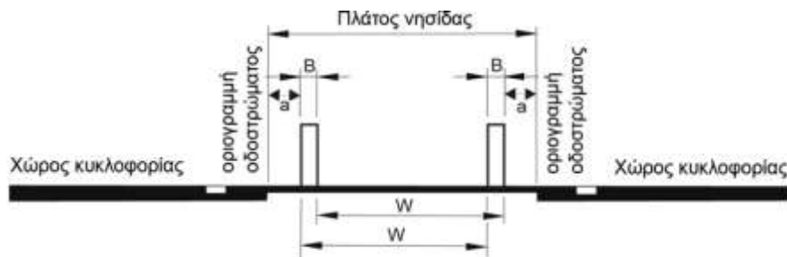
Μονόπλευρα μόνιμα στηθαία ασφαλείας με χωριστή δράση (και στις 2 οριογραμμές)
