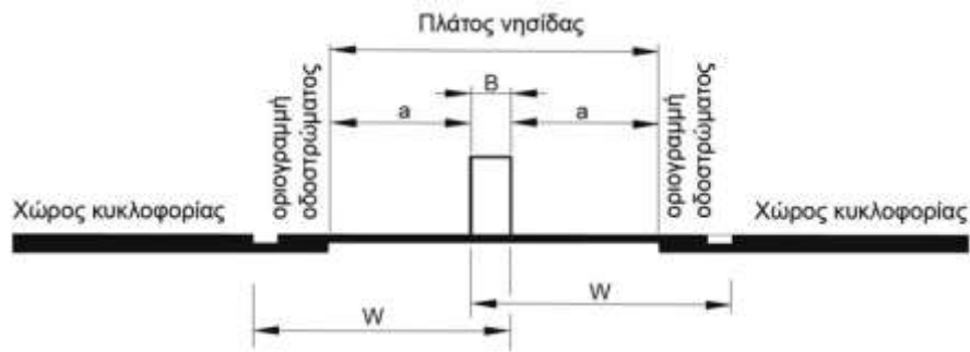
Αμφίπλευρο μόνιμο στηθαίο ασφαλείας που τοποθετείται στο μέσον της νησίδας
