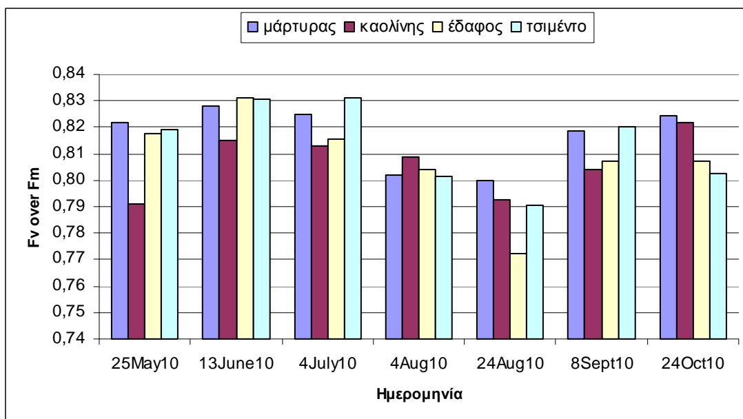
Διάγρ. 41. Μεταβολή του F_v/F_m , από το Μάιο έως τον Οκτώβριο, σε φύλλα ελιάς δένδρων με καρπούς που περιοδικά ψεκάστηκαν με νερό (μάρτυρας) ή με διάλυμα καολίνη 5% (καολίνης), ή εφαρμόστηκε κόνις εδάφους (έδαφος) ή κόνις τσιμέντου (τσιμέντο) ( E_{SD_{0,05}} = 0,028 ).
