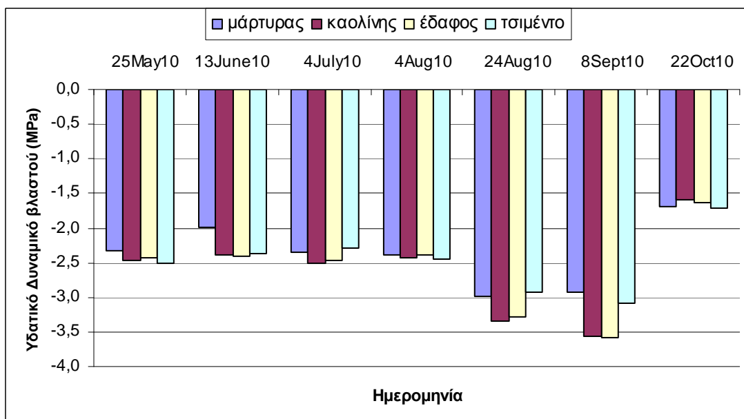
Διάγρ. 42. Μεταβολή του υδατικού δυναμικού βλαστού, από το Μάιο έως τον Οκτώβριο, σε φύλλα ελιάς δένδρων με καρπούς που περιοδικά ψεκάστηκαν με νερό (μάρτυρας) ή με διάλυμα καολίνη 5% (καολίνης), ή εφαρμόστηκε κόνις εδάφους (έδαφος) ή κόνις τσιμέντου (τσιμέντο) ( E\bar{S}\Delta_{0,05} = 3,34 ).
