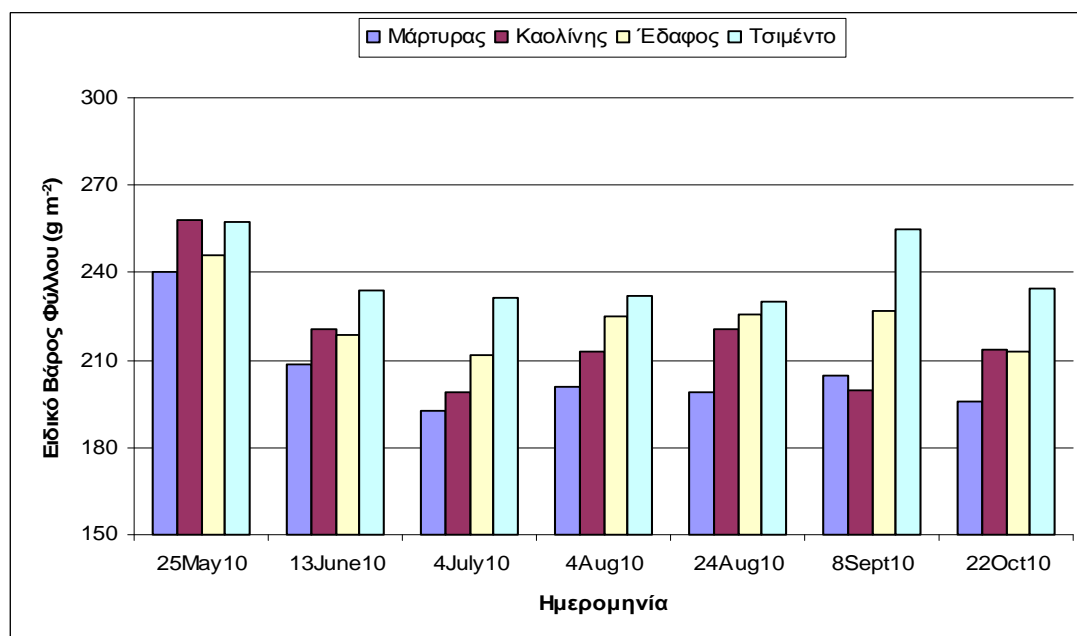
Διάγρ. 24. Μεταβολή του ειδικού βάρους φύλλου από τέλη Μαΐου μέχρι τέλη Οκτωβρίου σε φύλλα ελιάς δένδρων με καρπούς που περιοδικά ψεκάστηκαν με νερό (μάρτυρας) ή με διάλυμα καολίνης 5% (καολίνης), ή εφαρμόστηκε κόνις εδάφους (έδαφος) ή κόνις τσιμέντου (τσιμέντο) ( E\text{Σ}\Delta_{0,05} = 1,98 ).
