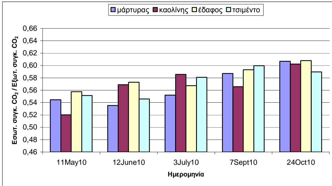
Διάγρ. 10. Μεταβολή της εσωτερικής συγκέντρωσης CO 2 προς εξωτερική συγκέντρωση CO 2 , από το Μάιο έως τον Οκτώβριο, σε φύλλα ελιάς δένδρων χωρίς καρπούς που περιοδικά ψεκάστηκαν με νερό (μάρτυρας) ή με διάλυμα καολίνη 5% (καολίνης), ή εφαρμόστηκε κόνις εδάφους (έδαφος) ή κόνις τσιμέντου (τσιμέντο) (ΕΣΔ 0,05 = 0,036).
