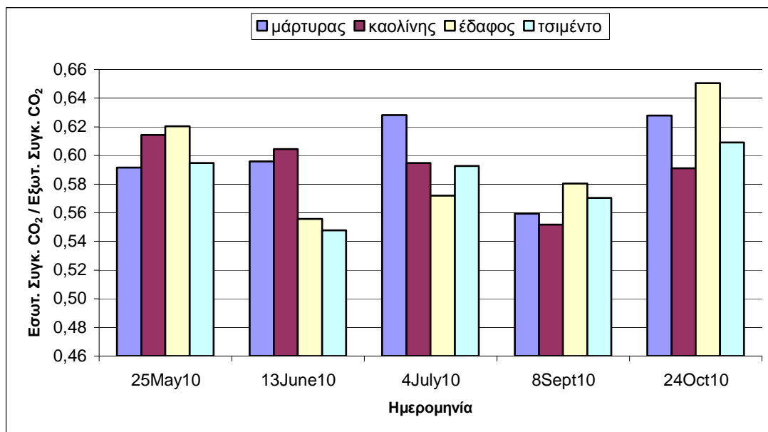
Διάγρ. 31. Μεταβολή της εσωτερικής συγκέντρωσης CO 2 προς εξωτερική συγκέντρωση CO 2 , από το Μάιο έως τον Οκτώβριο, σε φύλλα ελιάς δένδρων με καρπούς που περιοδικά ψεκάστηκαν με νερό (μάρτυρας) ή με διάλυμα καολίνη 5% (καολίνης), ή εφαρμόστηκε κόνις εδάφους (έδαφος) ή κόνις τσιμέντου (τσιμέντο) (ΕΣΔ 0,05 = 0,036).
