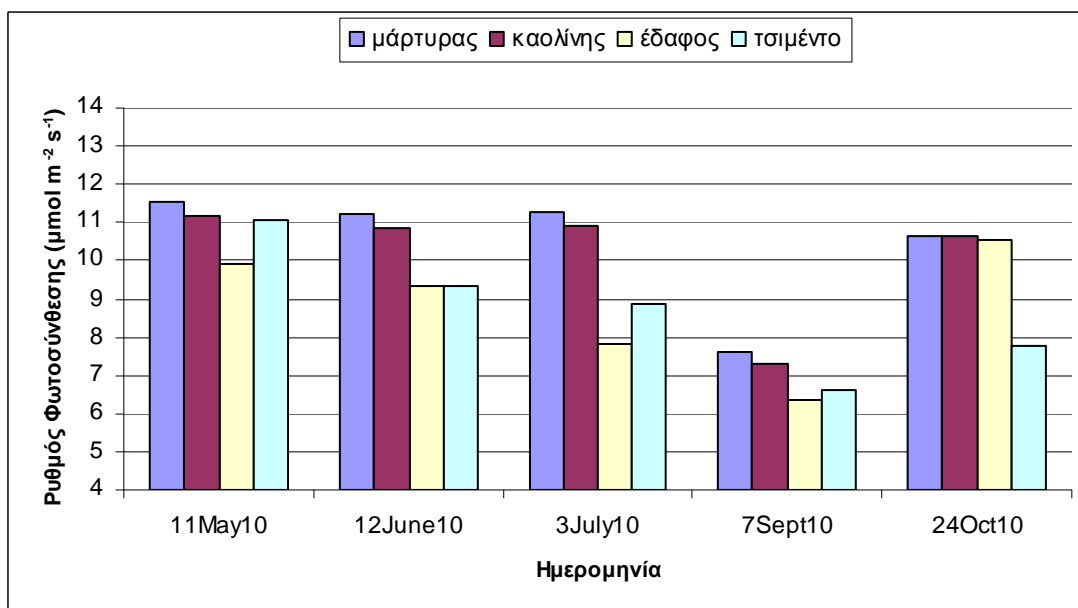
Διάγρ. 15. Μεταβολή του ρυθμού φωτοσύνθεσης, από το Μάιο έως τον Οκτώβριο, σε φύλλα ελιάς δένδρων χωρίς καρπούς που περιοδικά ψεκάζτηκαν με νερό (μάρτυρας) ή με διάλυμα καολίνη 5% (καολίνης), ή εφαρμόστηκε κόνις εδάφους (έδαφος) ή κόνις τσιμέντου (τσιμέντο) ( E\sigma\Delta_{0,05} = 1,27 ).
