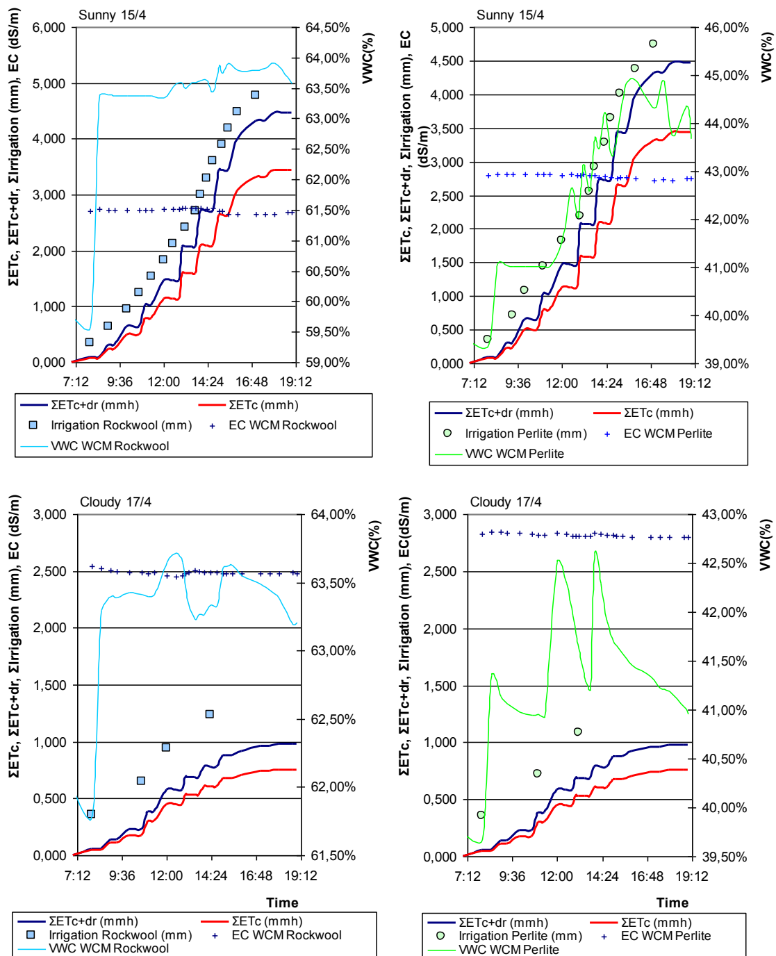
Εικόνα 78 Ημερήσια πορεία της εξαμισοδιαπνοής, της απαίτησης νερού (εξαμισοδιαπνοή και απορροή), της παροχής νερού, της υγρασίας υποστρώματος και της EC για δύο χαρακτηριστικές ημέρες (μία ηλιόλουστη (15/4) και μία νεφосκεπή (17/4)) κατά την δεύτερη περίοδο άρδευσης (αυτόματος προγραμματισμός με βάση την ηλιακή ακτινοβολία).
