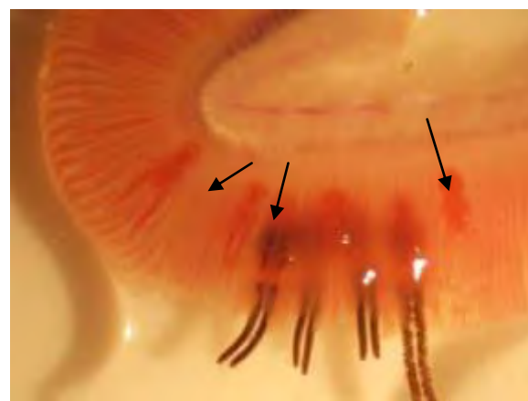
Εικ. 6.2 Αρσενικά (βέλη) και ωφόρα Θηλυκά Lernanthropus kroyeri
