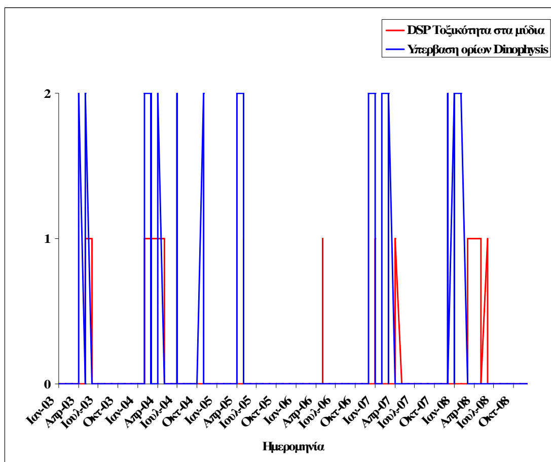
Εικόνα 6.69. Χρονικές περιόδους και αιτιολογία άρσης και λήψης υγειονομικών μέτρων των DSP τοξικών επεισοδίων κατά τα έτη 2003-2008 στο σημείο δειγματοληψίας Καβούρα (Θ6/M6) της νομαρχίας Θεσσαλονίκης.
