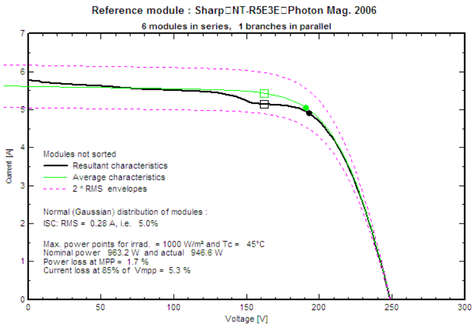
Διάγραμμα 3.2: Μέγιστη αποδιδόμενη ισχύς συστοιχίας που αποτελείται από 6 όμοια πάνελ συνδεδεμένα σε σειρά.
