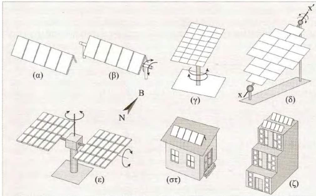
Εικόνα 2.8: (α) Τοποθέτηση ΦΒ συστοιχίας με σταθερή γωνία κλίσης (β) Συστοιχία με δυνατότητα στροφής γύρω από οριζόντιο άξονα (αλλαγή ζενιθίας γωνίας της συστοιχίας) (γ) Συστοιχία σε ηλιοτρόπιο αξιμουθιακής στροφής, με σταθερή γωνία κλίσης (δ) Συστοιχία με δυνατότητα στροφής ως προς τον άξονα (χχ'), ο οποίος διατηρείται κεκλιμένος συνήθως υπό γωνία ίση (ή μερικές φορές, λίγο μικρότερη) του γεωγραφικού πλάτους του τόπου, δηλαδή ως προς άξονα παράλληλο προς τον πολικό άξονα της γης. (ε) Τυπική διάταξη ηλιοτροπίου (Tracker) δύο αξόνων. (στ) ΦΒ συστοιχία στη στέγη κατοικίας (ζ) ΦΒ πλαίσια τοποθετημένα σε διάφορες θέσεις σε μεγάλη οικοδομή (τοποθέτηση υπό κλίση στη στέγη και σε προβόλους και κατακόρυφα (facade) σε όψεις νότιου προσανατολισμού).
