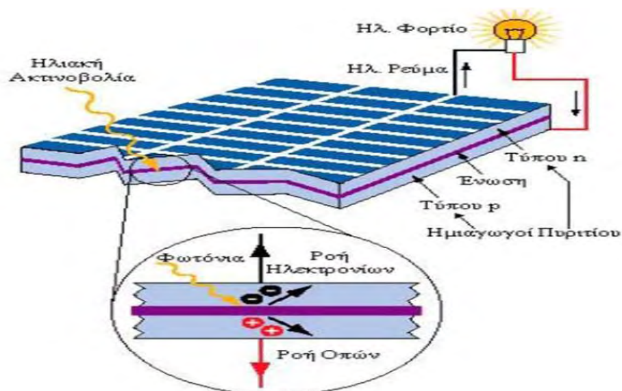
Εικόνα 1.1: Φωτοβολταϊκό φαινόμενο
