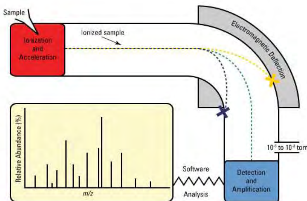
Εικόνα 15: Ένα δείγμα εγχέεται μέσα στο φασματόμετρο μάζας, και τα μόρια ιονίζονται και επιταχύνονται. Τα ιόντα στη συνέχεια διαχωρίζονται κατά μάζα και φορτίο από τον αναλυτή μάζας μέσω ηλεκτρομαγνητικής εκτροπής, και τα ιόντα τα οποία είναι κατάλληλα ευθυγραμμισμένα ανιχνεύονται και ενισχύονται. Το όλο σύστημα είναι υπό κενό κατά τη διάρκεια της όλης διαδικασίας. Μετά την ενίσχυση του σήματος από τους ανιχνευτές, τα «χτυπήματα» των ιόντων αναλύονται, και τα δεδομένα που δημιουργούνται, απεικονίζονται ως προς τη σχετική αφθονία του κάθε ιόντος με βάση τον λόγο μάζας προς φορτίο (Hoofmann and Stroobant, 2001).
