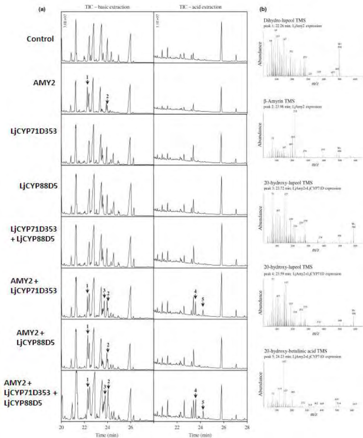
Εικόνα 18: Ανάλυση GC-MS των σαπωνοποιημένων εκχυλίσματων φύλλων του N. Benthamiana μετά την παροδική έκφραση των AMY2 , LjCYP71D353 ή/και LjCYP88D5 . (a): Συνολικά ιοντικά χρωματογραφήματα των παραγόμενων δειγμάτων από βασικά και όξινα εκχυλίσματα των φύλλων. Η έκφραση του γονιδίου AMY2 οδήγησε στην παραγωγή διυδρολουπεόλης (κορυφή 1) και \beta -αμυρίνης (κορυφή 2). Η συνδυαστική έκφραση των γονιδίων AMY2 και LjCYP71D353 οδήγησε στην παραγωγή της 20-υδροξυλουπεόλης (κορυφή 3 με χρόνο κατακράτησης τα 23,7 λεπτά στα βασικά εκχυλίσματα και κορυφή 4 με χρόνο κατακράτησης τα 23,59 λεπτά στα όξινα εκχυλίσματα) και του 20-βετουλινικού οξέος (κορυφή 5, με χρόνο κατακράτησης τα 24,22 λεπτά κατά την όξινη εκχύλιση). Δεν παρατηρήθηκε κάποια δραστηριότητα του γονιδίου LjCYP88D5 . Οι υπόλοιπες κορυφές αντιστοιχούν στις φυτικές στερόλες. (b): Φάσματα μαζών των κορυφών 1-5 που προέρχονται από τα προφίλ της αέριας χρωματογραφίας του σχήματος (a).
