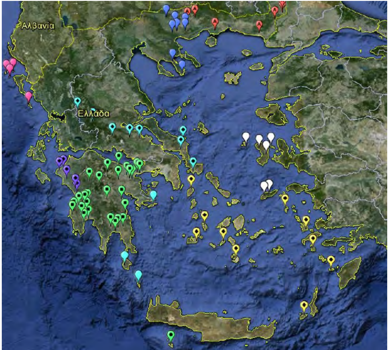
Χάρτης 3.1 Ενεργοί ΧΑΔΑ στην Ελλάδα (2013) (πηγή: http://www.ypeka.gr )
