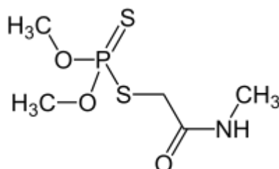
Εικόνα 3. Χημικός τύπος του dimethoate.
