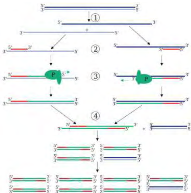
Εικόνα 6. Σχηματική απεικόνιση του κύκλου της PCR (1) Αποδιάταξη στους 94-96 o C. (2) Υβριδισμός στους (π.χ.) 68 o C. (3) Επιμήκυνση στους 72 o C (P=Polymerase=Πολυμεράση). (4) Ο πρώτος κύκλος έχει ολοκληρωθεί. Οι δύο νέοι κλώνοι θα αποτελέσουν το εκμαγείο για τον επόμενο κύκλο, διπλασιάζοντας έτσι την ποσότητα του DNA που αντιγράφεται σε κάθε νέο κύκλο.
