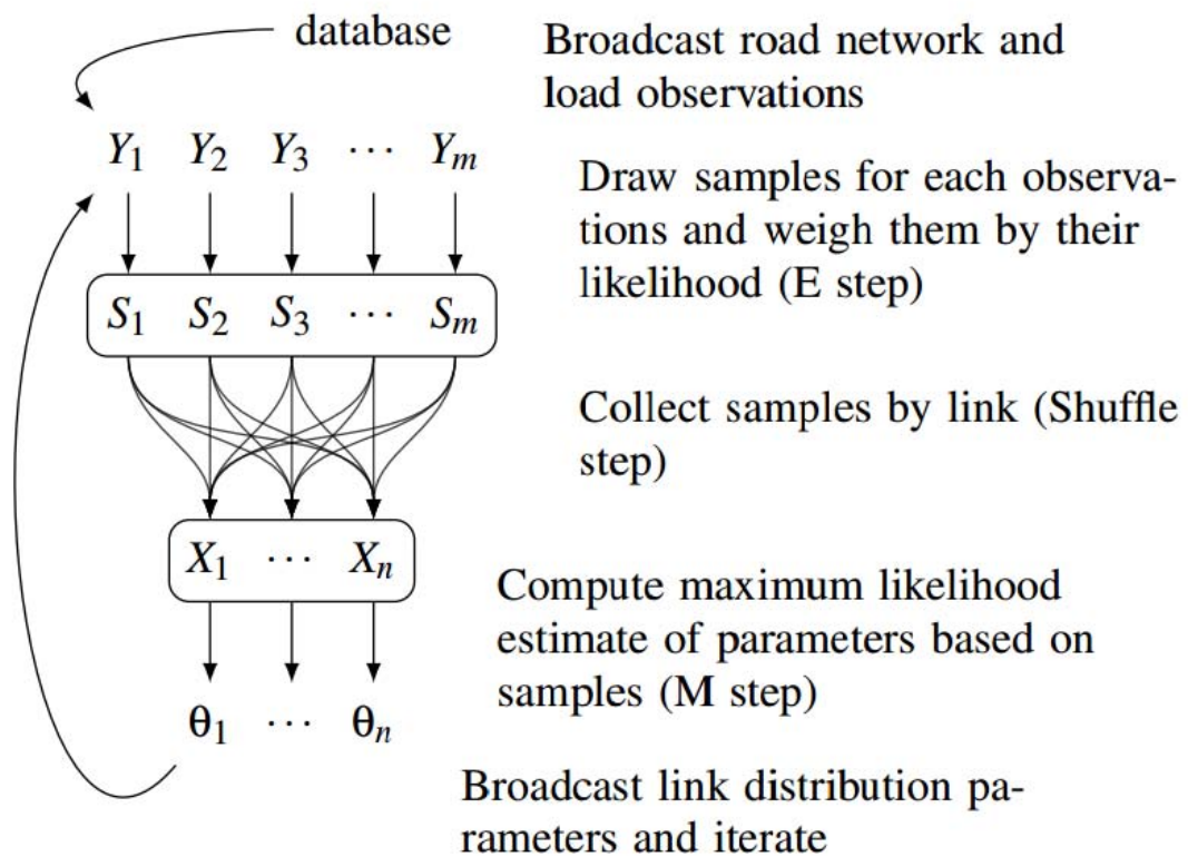
ΣΧΗΜΑ 7.5: Διάγραμμα ροής της λειτουργίας του EM αλγορίθμου [21].
