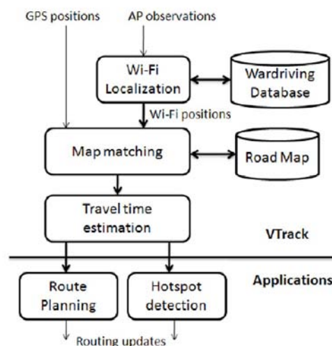
ΣΧΗΜΑ 6.3: Λειτουργία του εξυπηρετητή [3].
