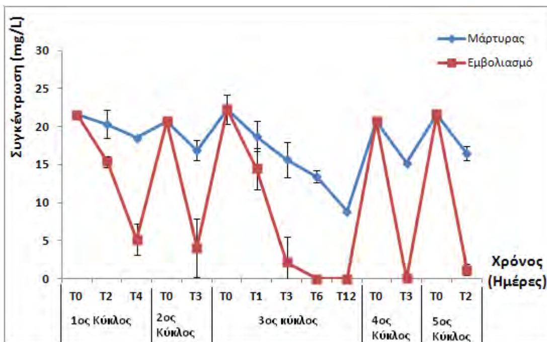
Διάγραμμα 3. Η αποδόμηση του οξαμυλ στους πέντε κύκλους εμπλουτισμού σε θρεπτικό μέσο MSM και σε μη εμβολιασμένο θρεπτικό μέσο MSM (control). Κάθε τιμή αποτελεί το μέσο όρο τριών επαναλήψεων \pm τυπική απόκλιση.
