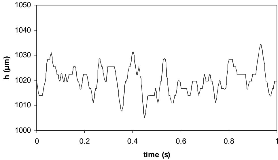
Σχήμα 3.4 Χρονική εξέλιξη πάχους υγρής στιβάδας για σύστημα νερού-αέρα σε u_{GS}=6.6 m/s και u_{LS}=0.002 m/s
