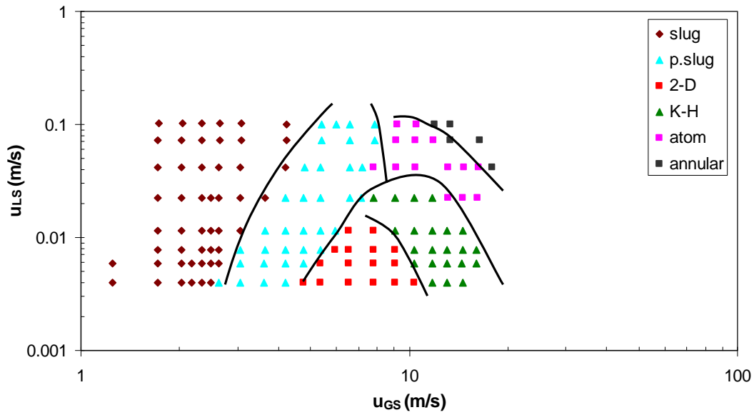
Σχήμα 8.6 Χάρτης καθεστώτων ροής για σύστημα νερού-CO 2 σε \varphi=1^\circ
