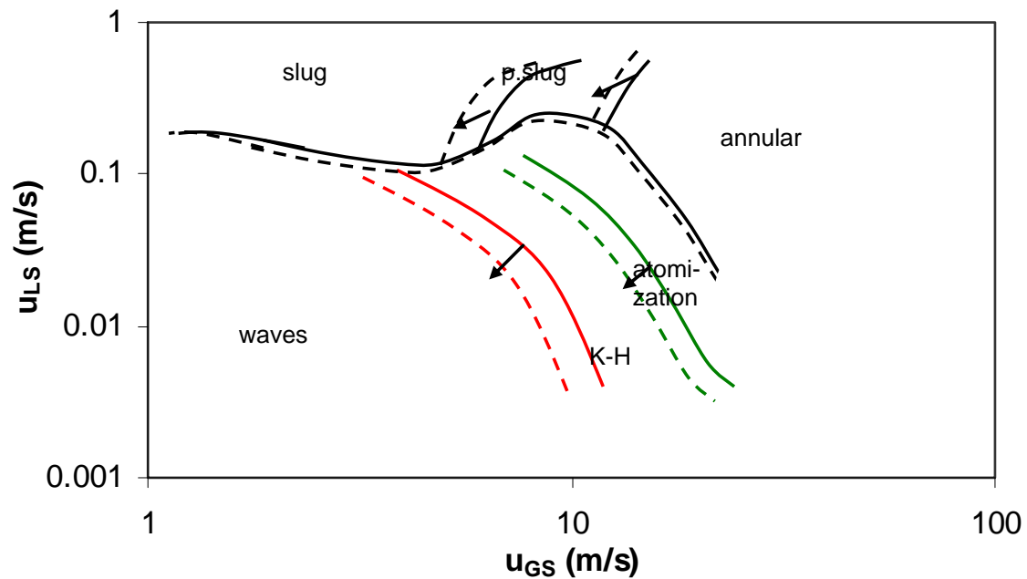
Σχήμα 7.11 Σύγκριση χαρτών ροής για το σύστημα νερού-αέρα (συνεχείς γραμμές) και υδατικού διαλύματος κανονικής βουτανόλης-αέρα σε κλίση \varphi=1^\circ (διακεκομμένες γραμμές)
