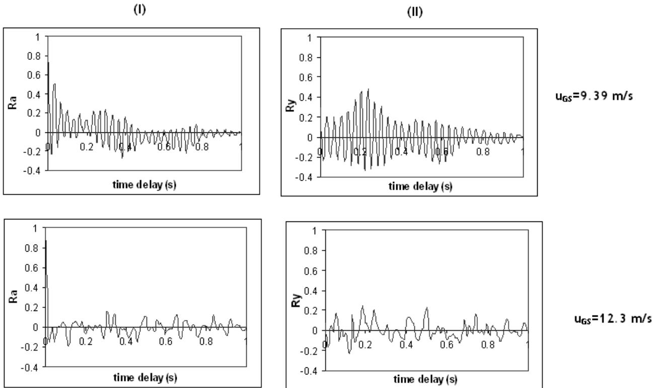
Σχήμα 8.20 Συναρτήσεις αυτοσυσχέτισης (I) και ετεροσυσχέτισης (II) για 2-D ( u_{GS}=9.4\text{m/s} ) και K-H κύματα ( u_{GS}=12.3 \text{ m/s} ) για σύστημα νερού-αέρα σε \varphi=0.25^\circ και u_{LS}=0.0078\text{m/s}
