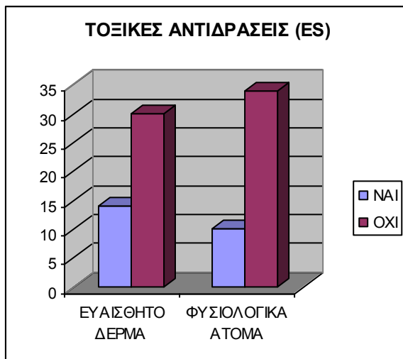
Εικόνα 6.1. και 6.2.: Συγκριτική μελέτη της εμφάνισης τοξικών αντιδράσεων στα αλλεργιογόνα της σειράς European standard (6.1.) και Cosmetics (6.2.), μεταξύ ασθενών με ευαίσθητο δέρμα και φυσιολογικών ατόμων.
