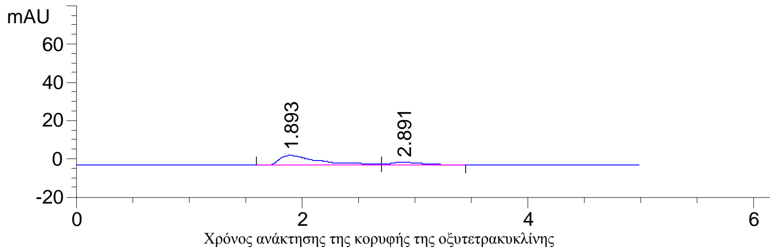
Σχήμα 19: Χρωματογράφημα 3 ου δείγματος ιχθυοτροφής με 4ml ιχθυέλαιο για εμφύσηση 2 min σε θαλασσινό νερό.
