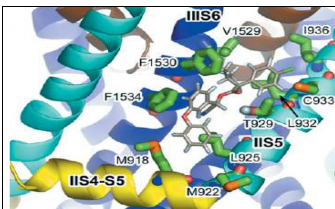
Εικόνα 2.8.: Θέσεις πρόσδεσης των πυρεθροειδών στο κανάλι Νατρίου της οικιακής μύγας (από O'Reilly et al., 2006)
