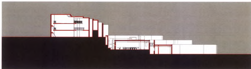
τομή 8
