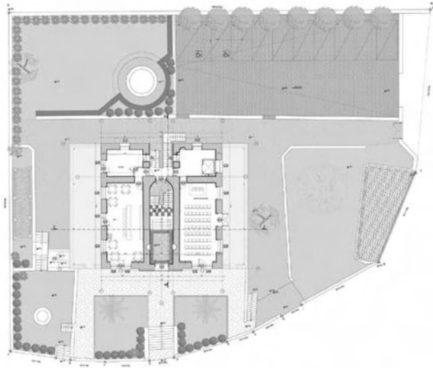
ΚΑΤΟΨΗ ΙΣΟΓΕΙΟΥ
