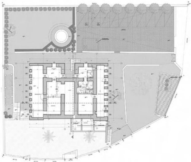
ΚΑΤΟΨΗ ΥΠΟΓΕΙΟΥ
